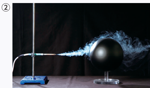
障害物を設置した場合のKOACH内部の気流の流れ
