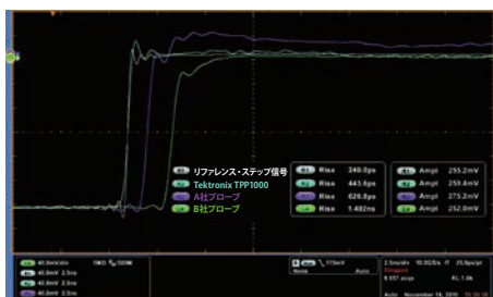
周波数帯域による影響
