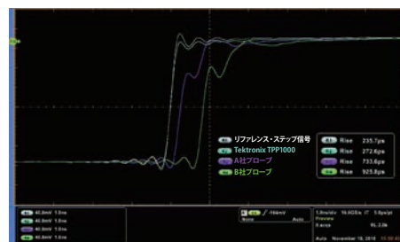
プローブ負荷による影響
